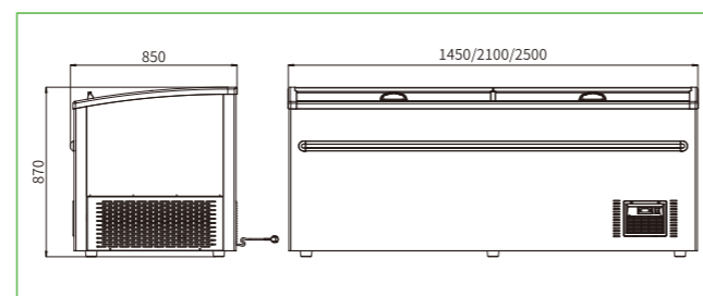
ZCD-L145S 侧柜
