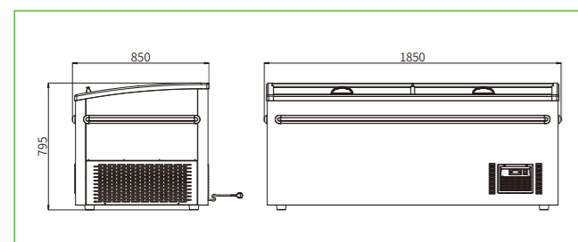
ZCD-E185S 端柜
