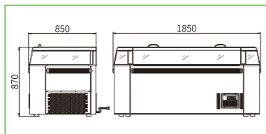
ZCD-E185S-S4 端柜
